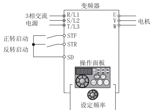
[接线例]
