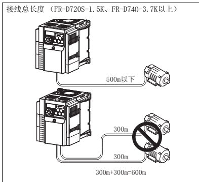
接线总长度 (FR-D720S-1.5K、FR-D740-3.7K以上)
