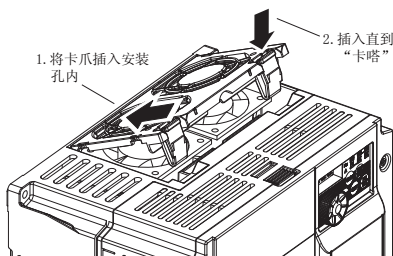
FR-D740-7.5K-CHT的示例
