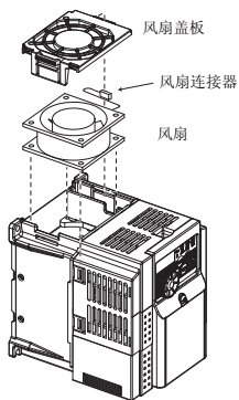
FR-D740-1.5K-CHT的示例
