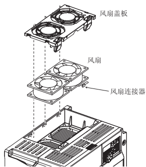
FR-D740-7.5K-CHT的示例
