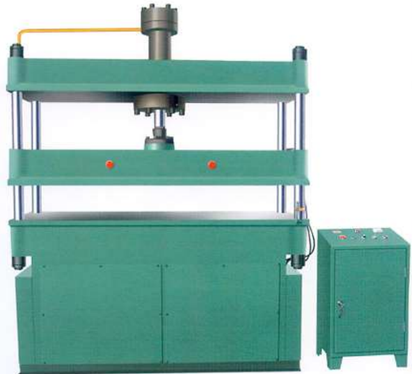
140吨油压平面式裁断机
